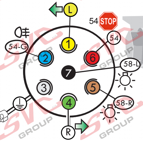
Pohled zezadu do zásuvky na upínací šroubky vodičů
